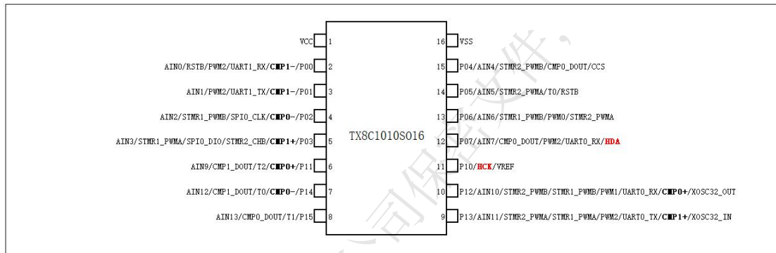
图 1-6 TX8C1010S016 (SOP16) 引脚图
