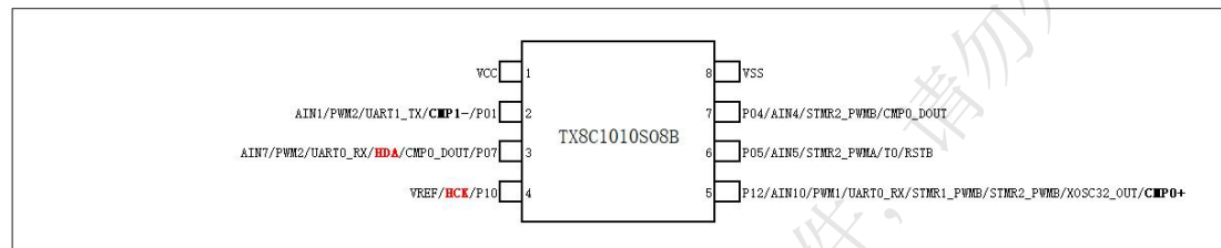
图 1-1 TX8C1010S08B（SOP8）引脚图
