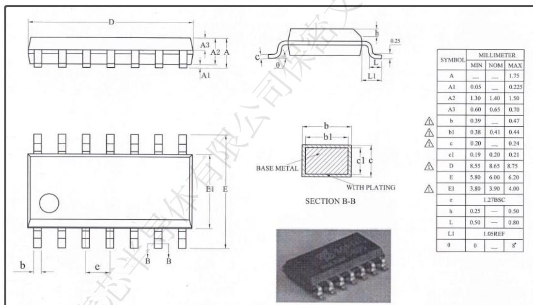
图 1-12 SOP14 封装 POD 图
