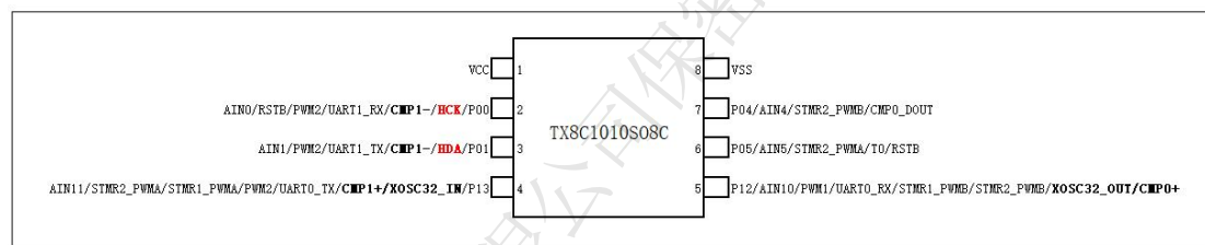
图 1-2 TX8C1010S08C（SOP8）引脚图
