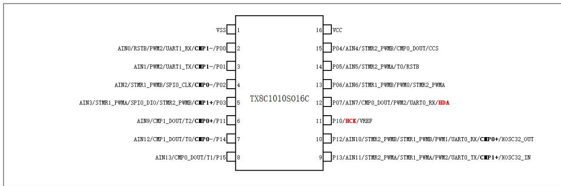
图 1-8 TX8C1010S016C (SOP16) 引脚图
