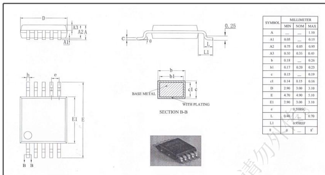
图 1-11 MSOP10 封装 POD 图
