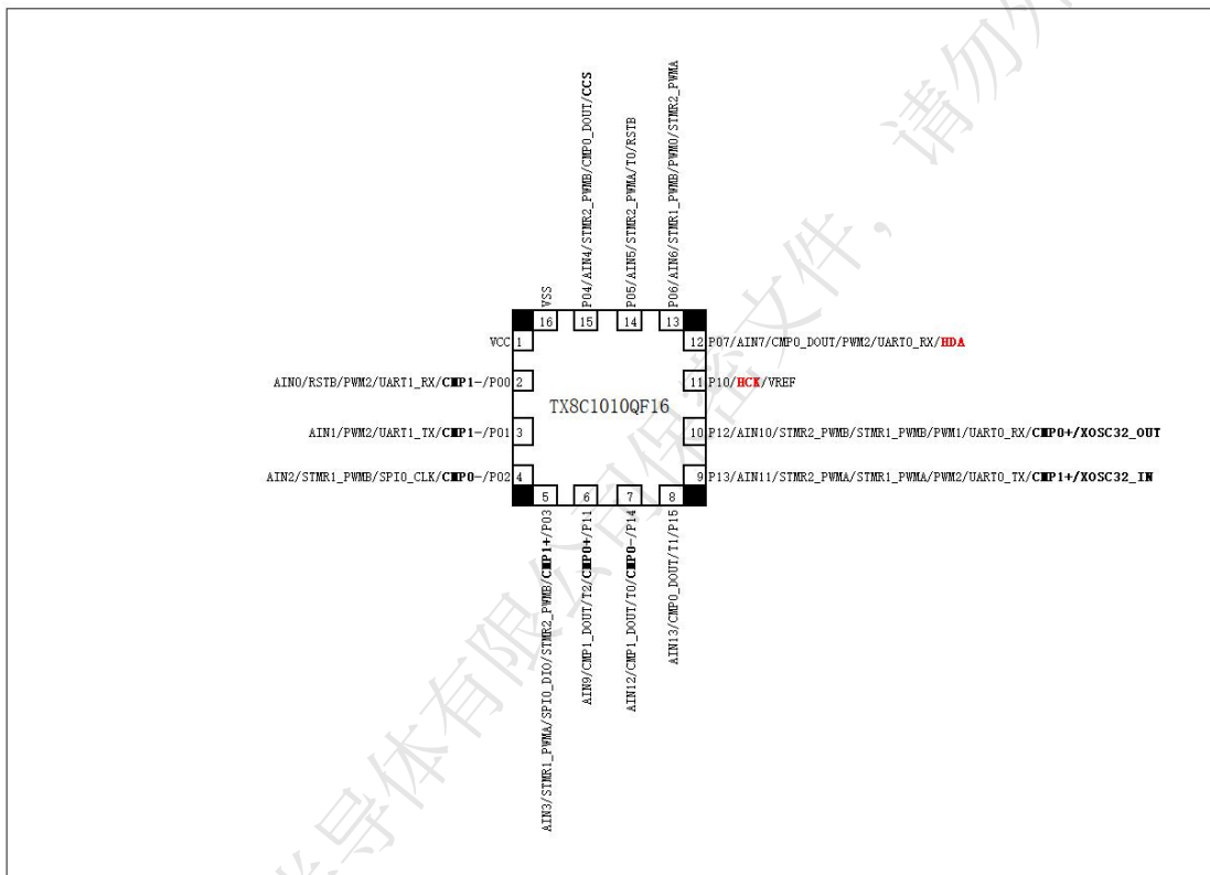
图 1-9 TX8C1010QF16 引脚图
