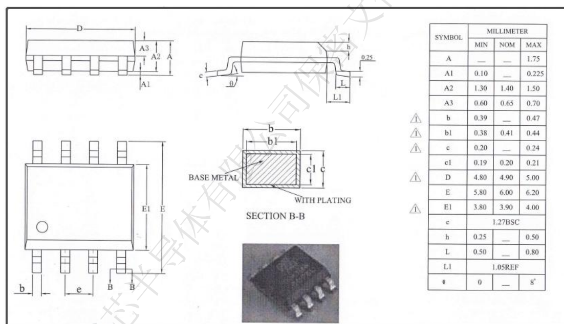
图 1-10 SOP8 封装 POD 图
