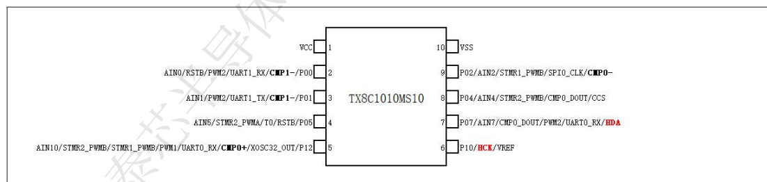
图 1-3 TX8C1010MS10（MSOP10）引脚图
