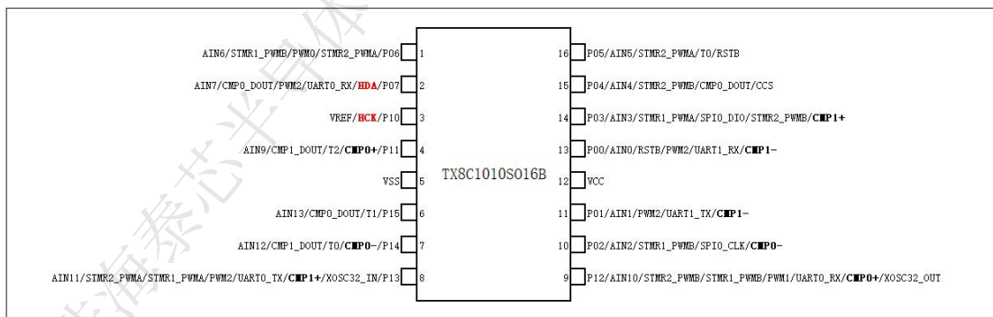
图 1-7 TX8C1010S016B (SOP16) 引脚图
