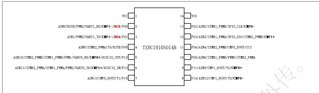
图 1-5 TX8C1010S014B (SOP14) 引脚图
