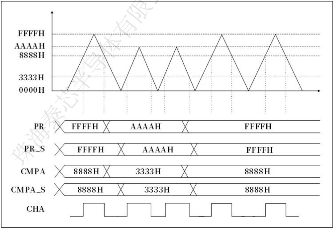
图 14-6 自动装载波形图
