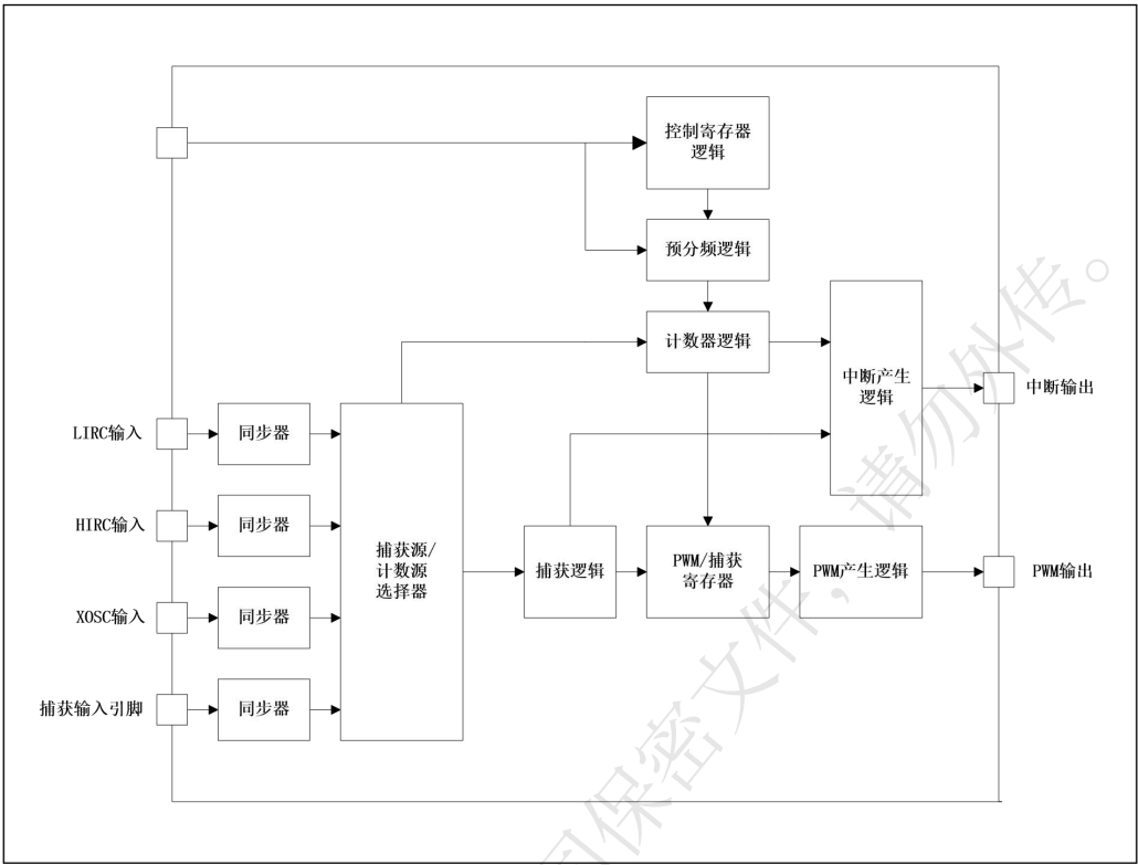
图 12-1 Timer0/1 模块框图
