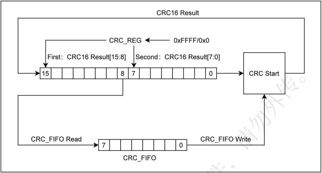
图 15-1 CRC16 结构框图
