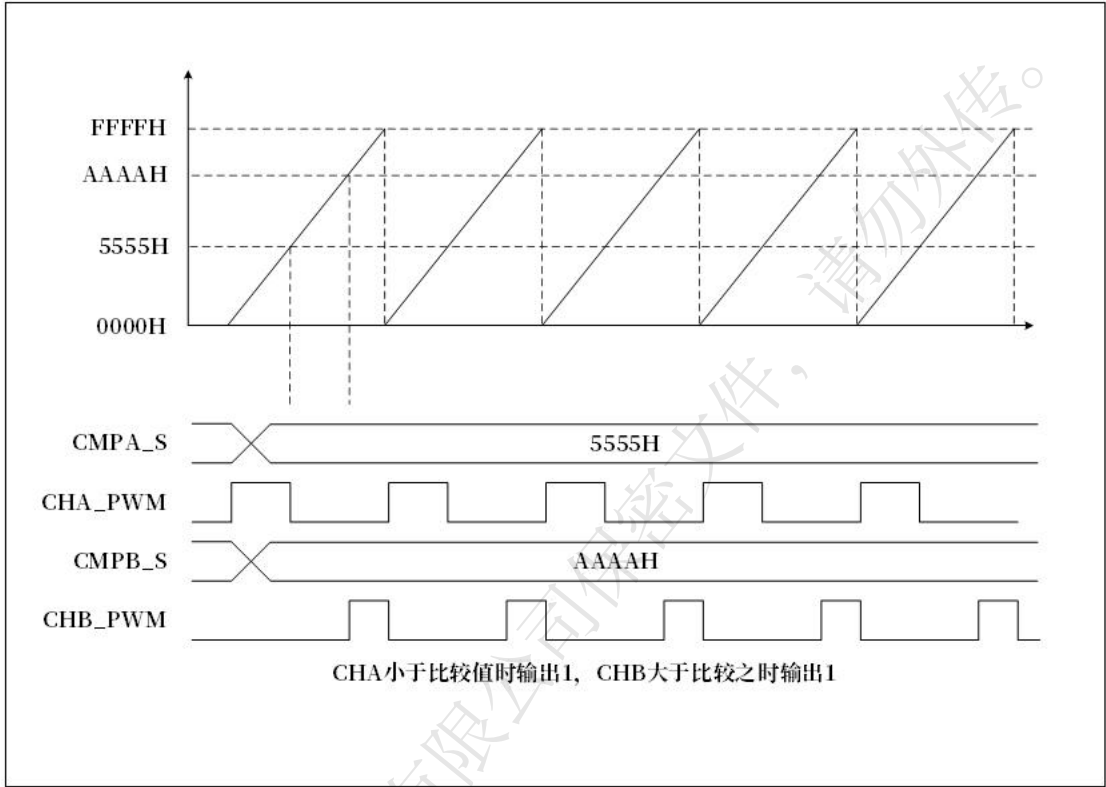
图 14-2 比较输出波形图
