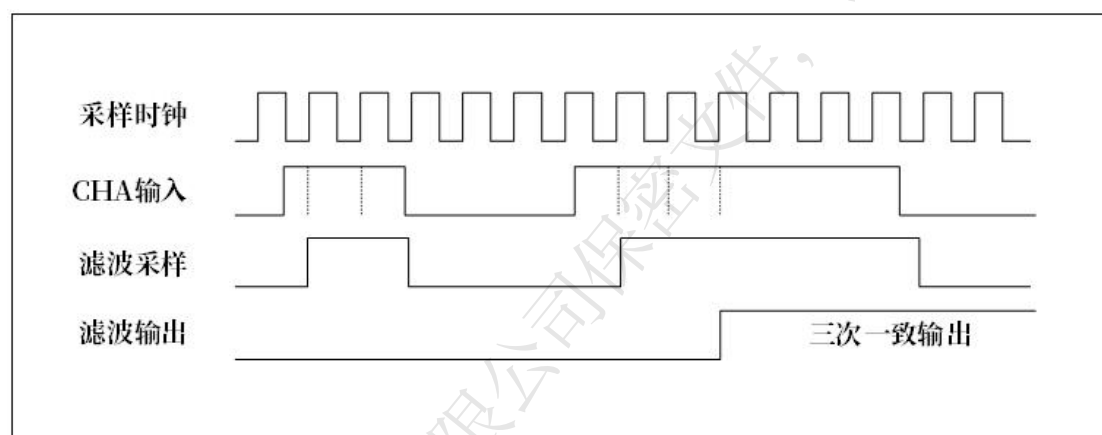
图 14-4 数字滤波波形图
