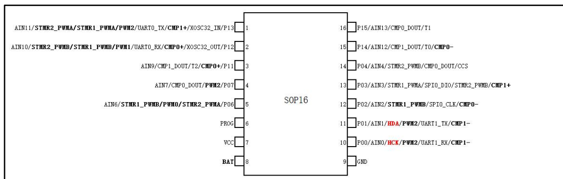
图 1-2 TX8P6010S016 引脚图
