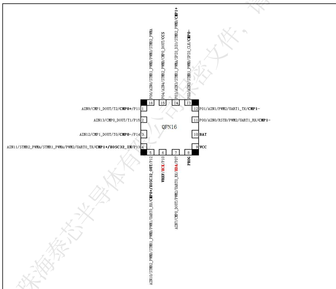
图 1-1 TX8P6010QF16 引脚图
