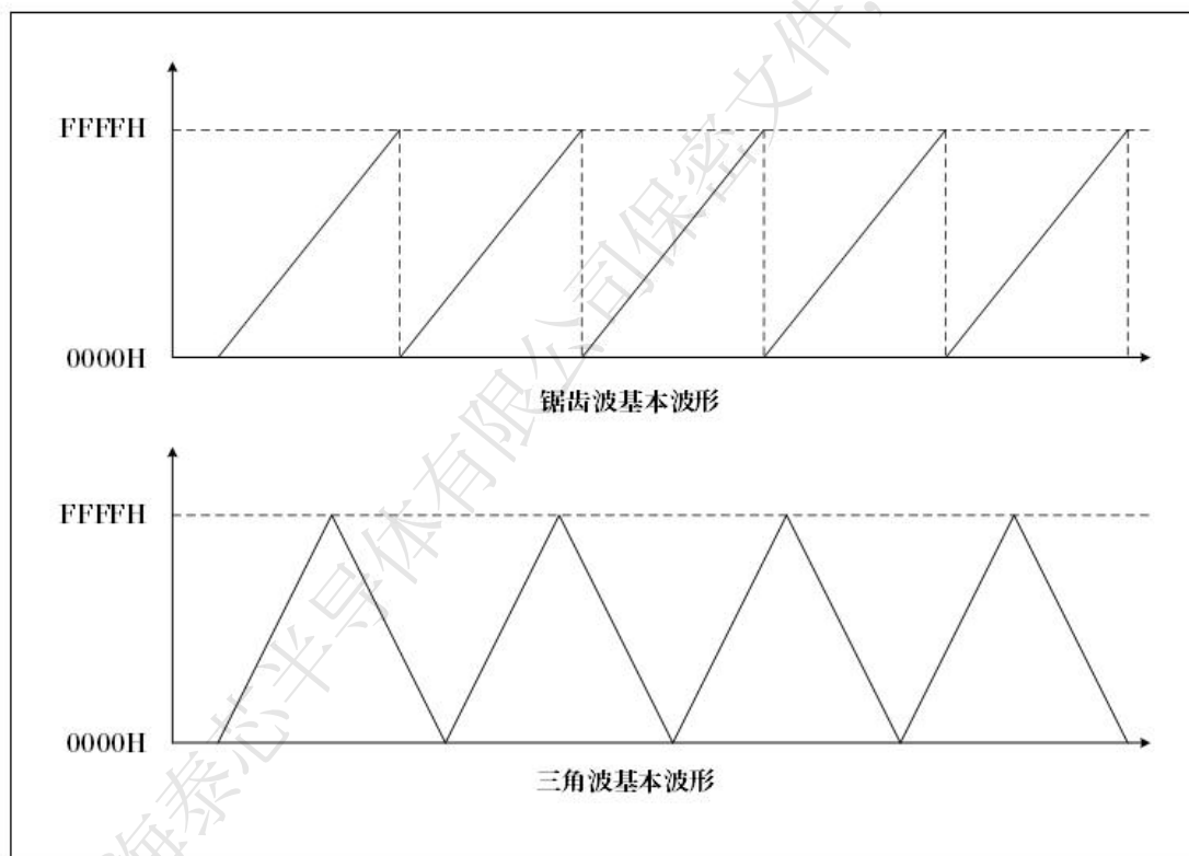
图 14-1 基础波形图
