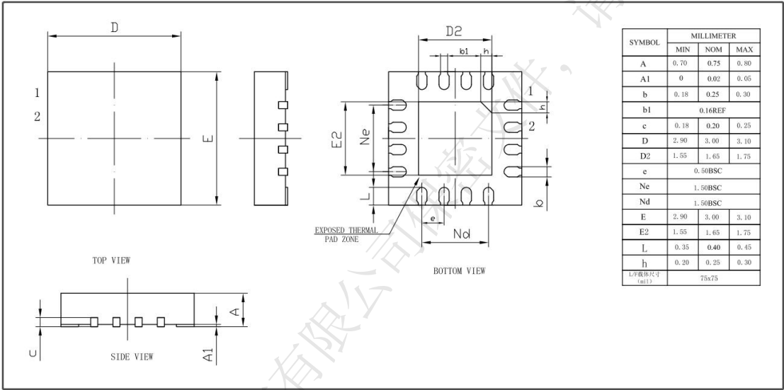
图 1-2 QFN16 封装 POD 图
