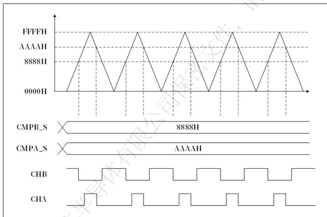
图 14-8 软件设定 CMPB_S 互补 PWM 波的示例
