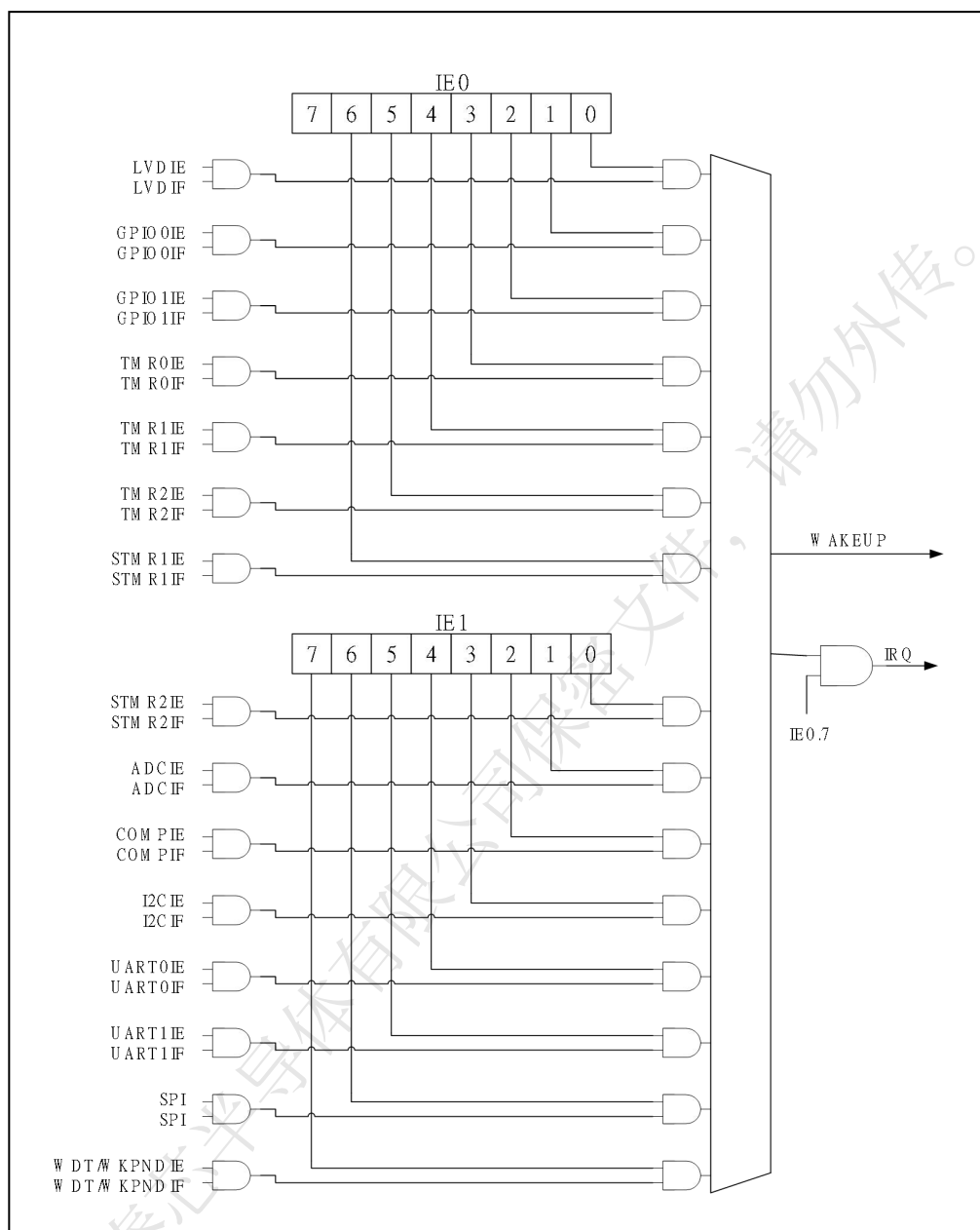
图 8-1 中断结构图
