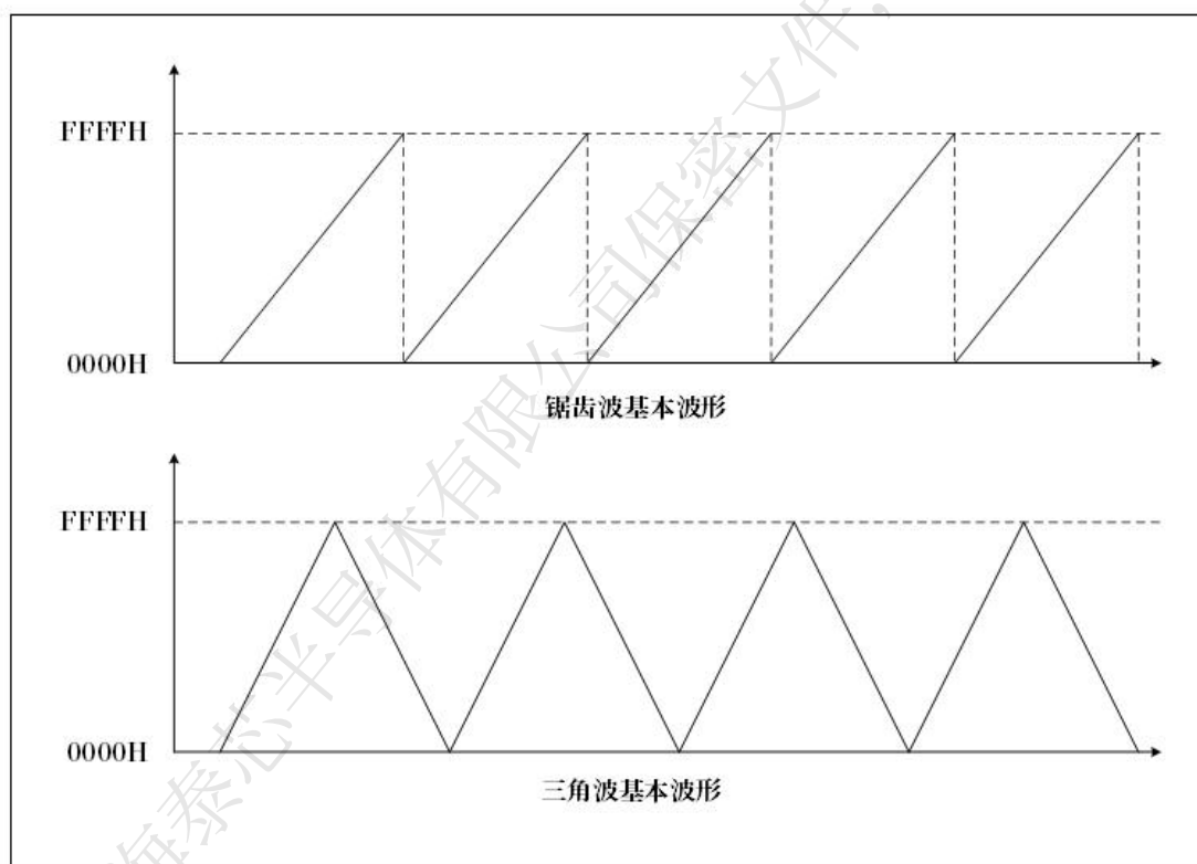
图 14-1 基础波形图
