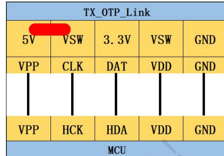
4 线仿真/烧录
