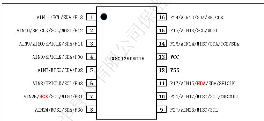
图 8 - TX8C1260S016 (SOP16) 封装图
