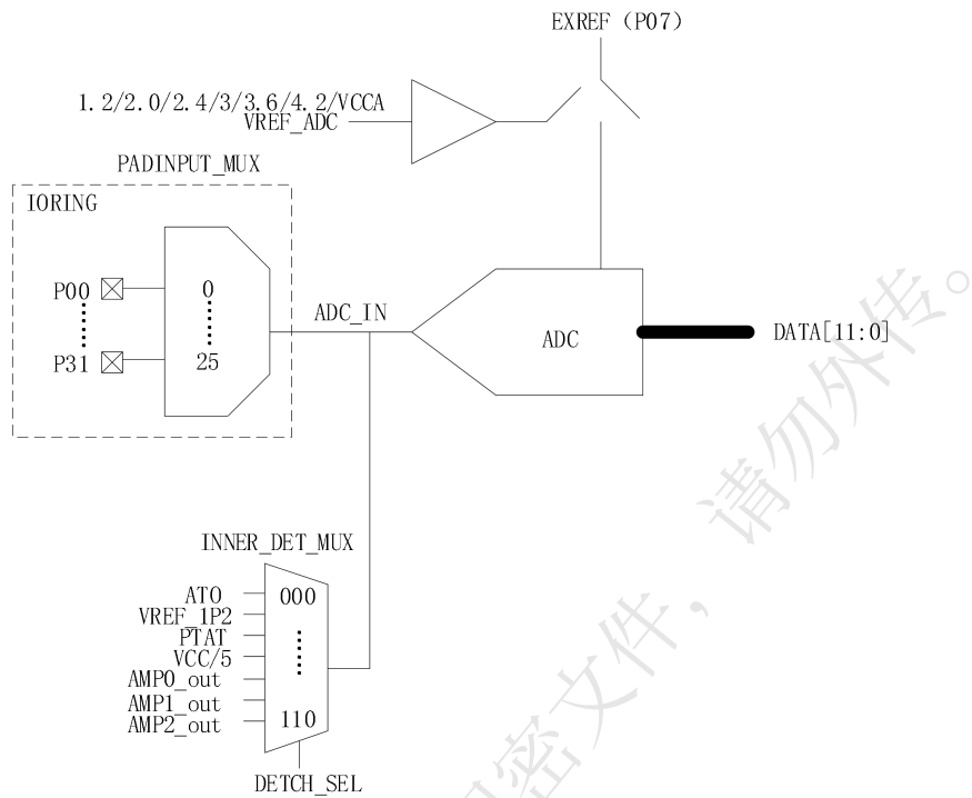
图 19- 5 ADC 模块结构框图
