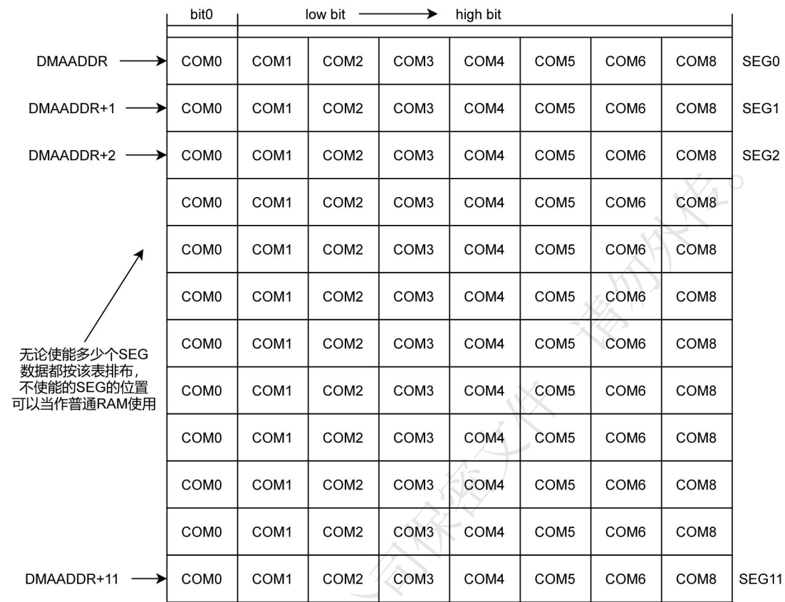
图 22- 3 SEG 扫描的数据结构
