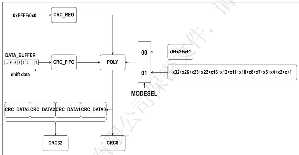
图 17- 1CRC 模块结构框图
