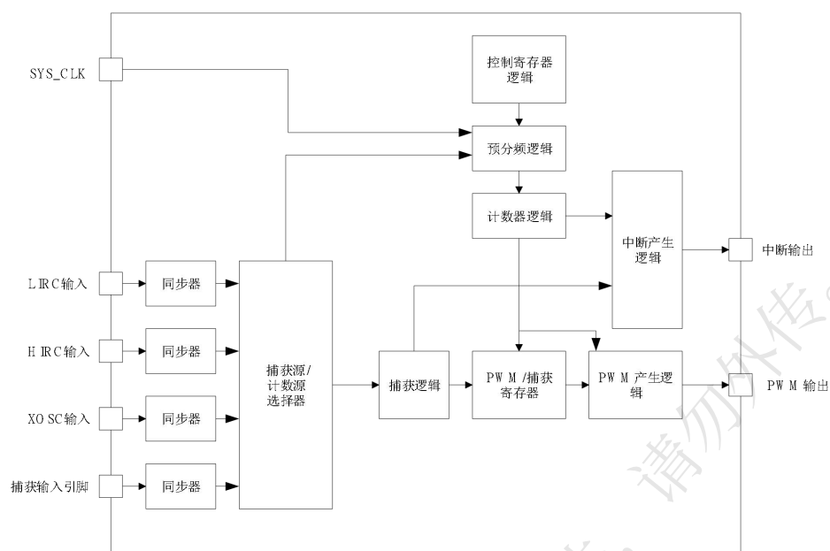
图 15- 3 Normal Timer 模块框图
