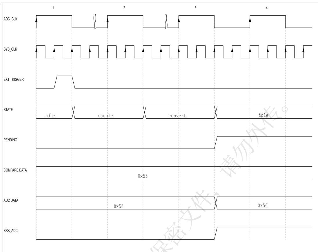
图 19-4 数字比较器模式工作时序图
