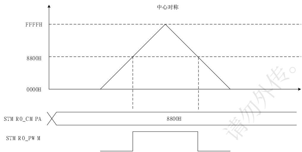
图 16- 4 PWM 中心对齐模式波形图
