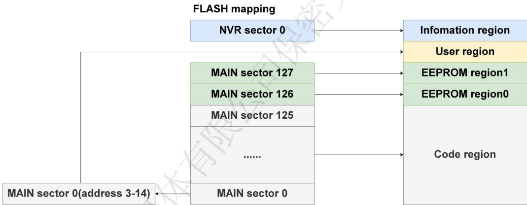
图 18-2 FLASH mapping 框图
