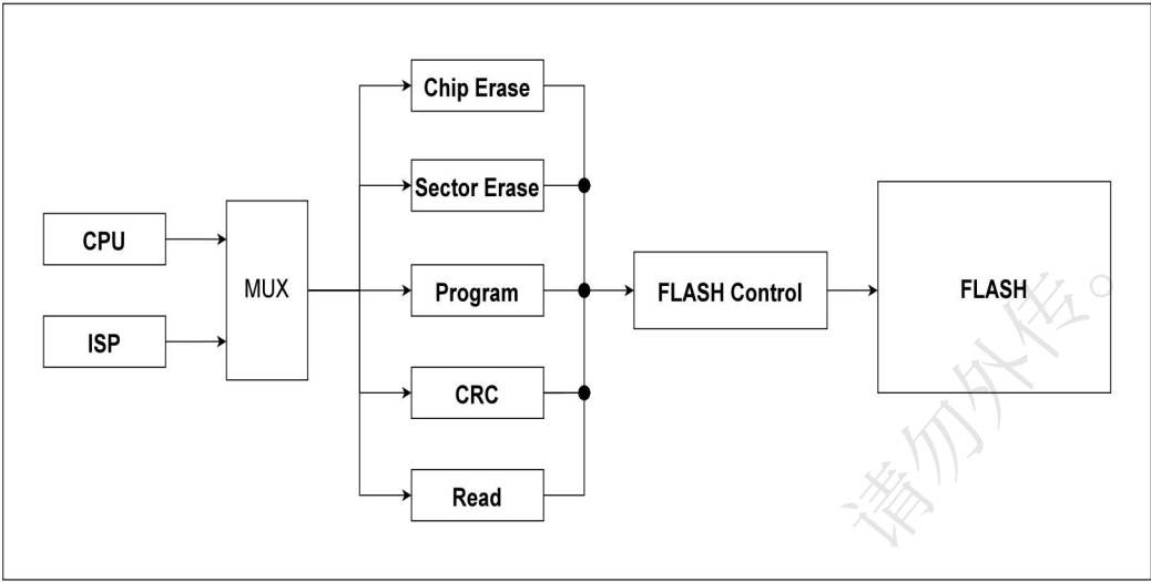
图 18-1 Flash 控制器模块框图
