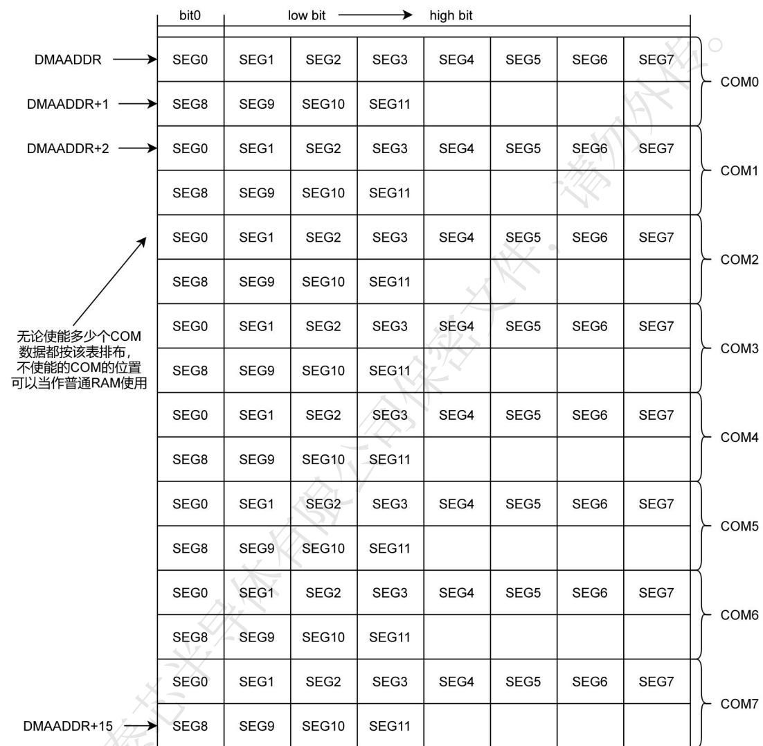
图 22- 2 COM 扫描的数据结构
