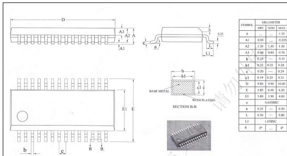
图 3- SSOP28 封装 POD 图
