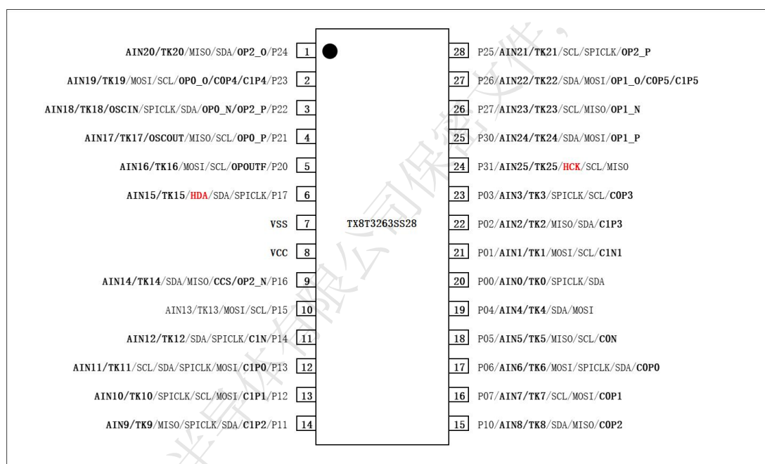
图 1 - TX8T3263SS28 (SSOP28) 封装图
