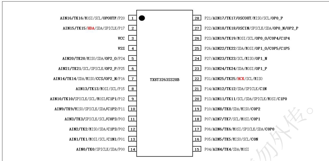
图 2 - TX8T3263SS28B (SSOP28) 封装图
