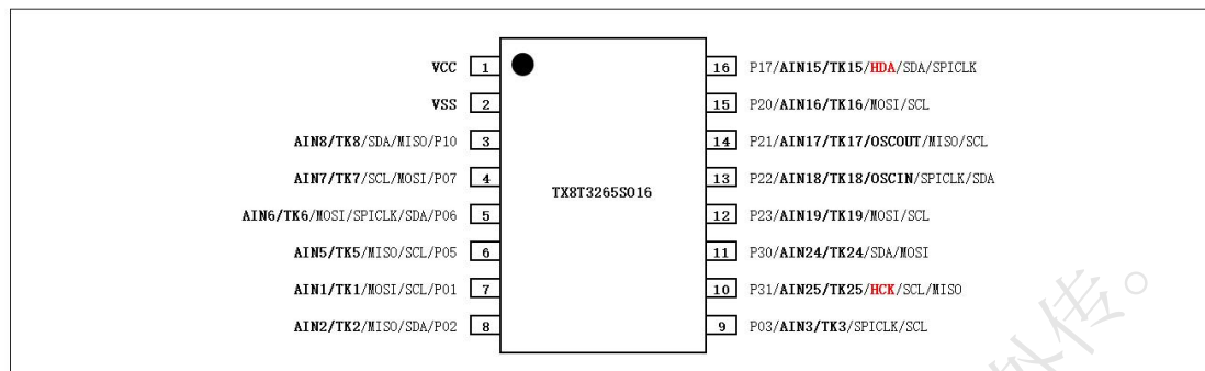
图 1 - TX8T3265S016 (SOP16) 封装图
