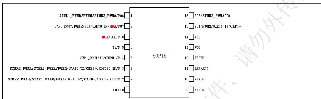
图 1-1 TX8W7010S016 引脚图
