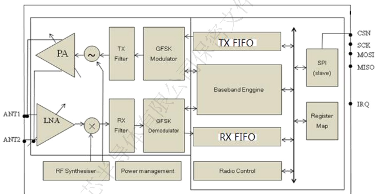
图-18.2 TX8W7010 RF 收发器模块系统结构框图
